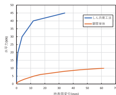
水平力と地表面変位の比較
